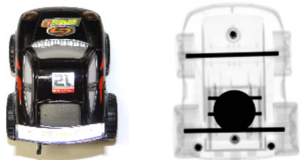
レントゲンで透過撮影した おもちゃの車
